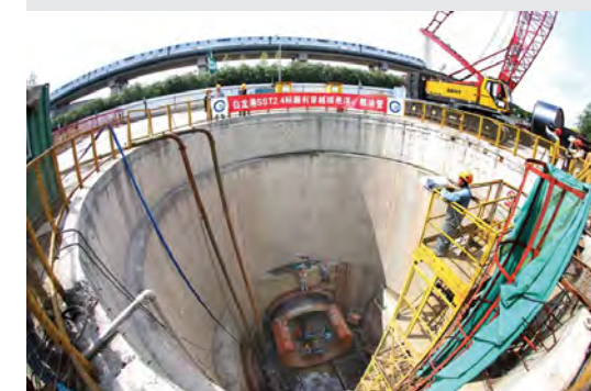
上海污水治理白龙港南线输送干线
